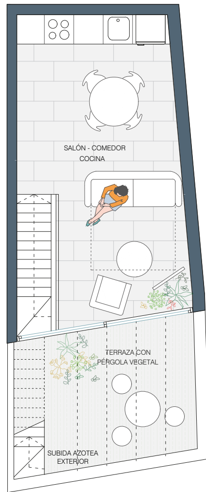
PLANTA ÁTICO
